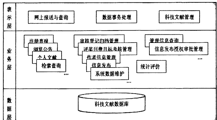
图1 在B/S架构中系统功能与各层次的对对应关系
